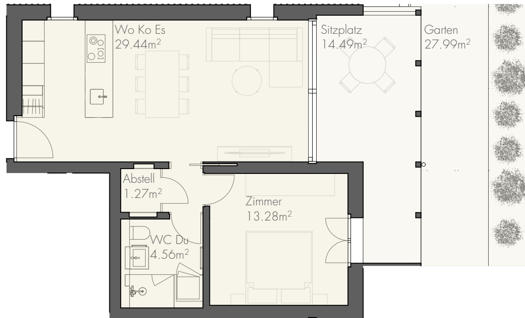
Erdgeschoss
